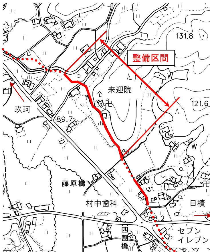
【右：伊陸久可地地区の整備予定位置図】
